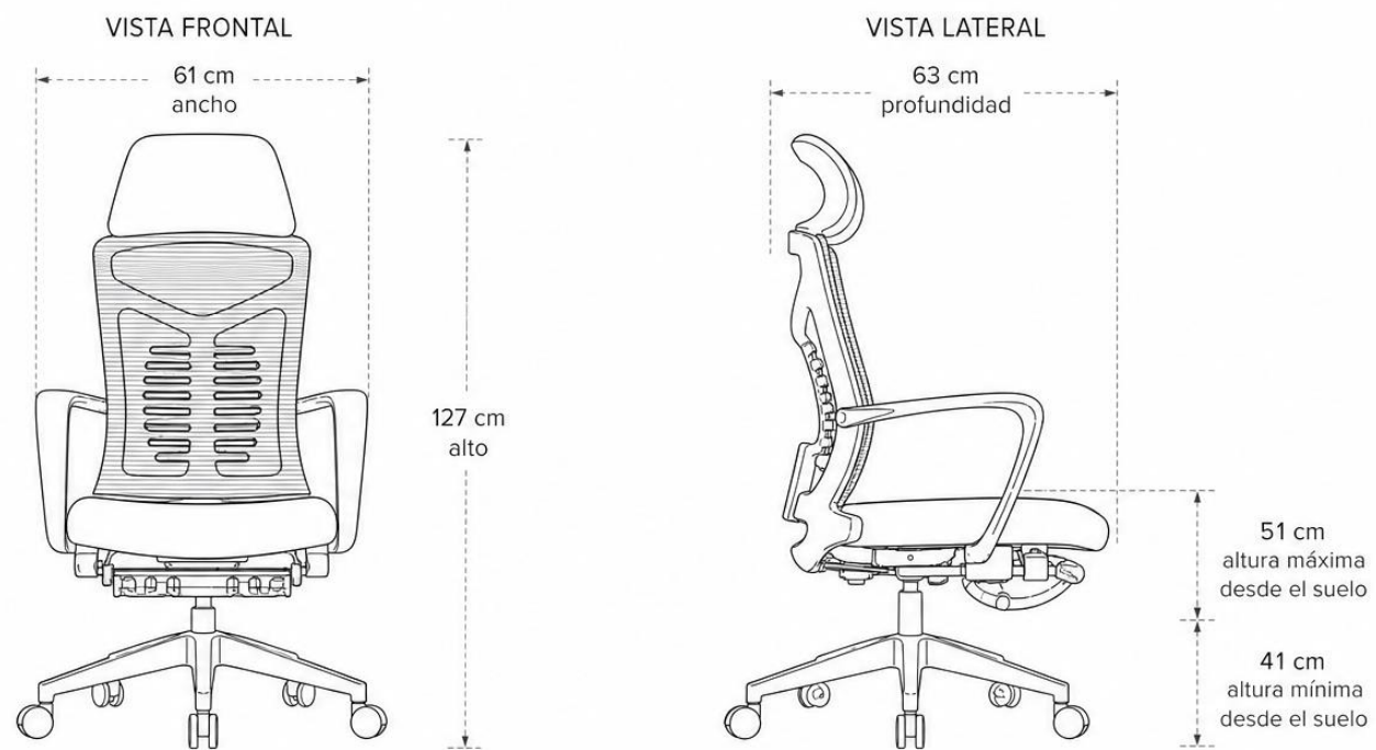
SILLA EJECUTIVA OPUS
