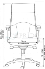
PLANO FRONTAL
