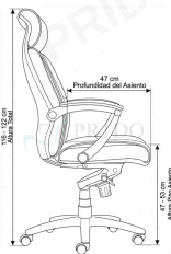
PLANO LATERAL
