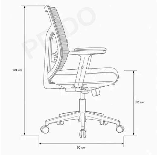
VISTA LATERAL
